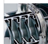
5 waaiers
