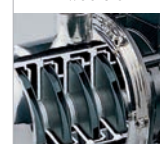
4 waaiers
