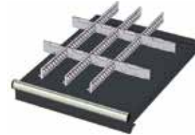
3x PROFILS DE SEPARATION 612mm 6x PROFILS CRANTES 102mm 2x PROFILS CRANTES 153mm
